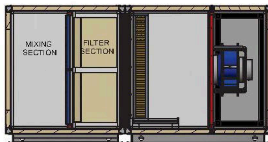
A-A ( 1 : 30 )
